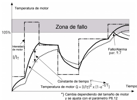
Figura 10.7: Cálculo de la temperatura del motor
